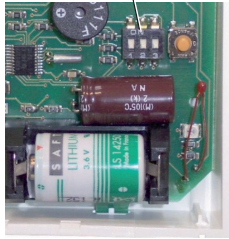
Funkfernbedienung(FFB)
