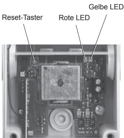
Empfängerteil
