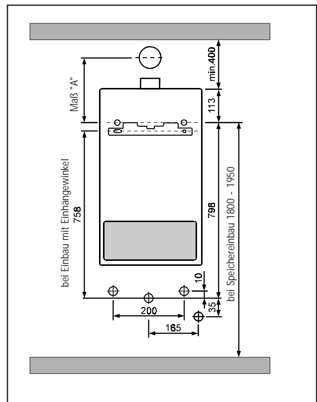
Bild: Einbaumaße
