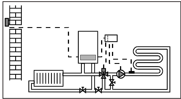
Bild: Fußbodenheizung
