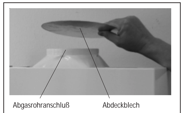
Bild: Abgasrohranschluß abdecken
