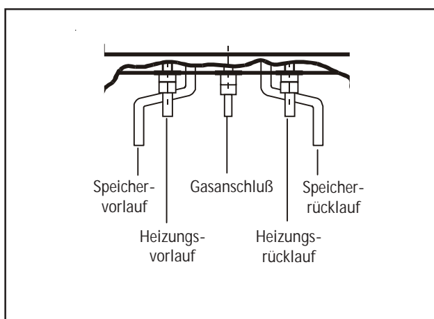
Bild: Anschlüsse GU-2E-S
