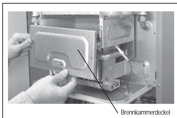
Bild: Brennkammerdeckel
