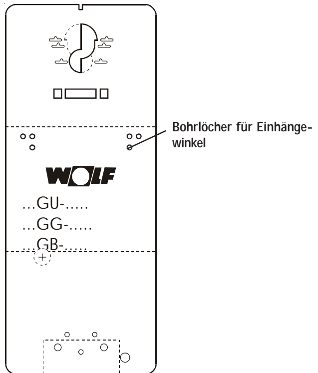
Bild: Einbauschablone
