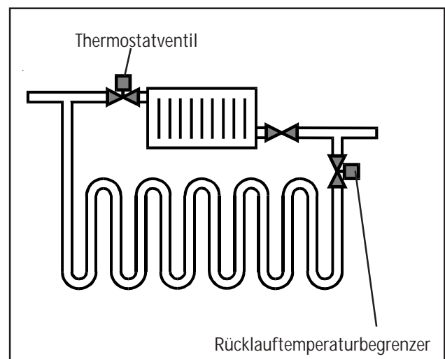
Bild: Fußbodenheizung
