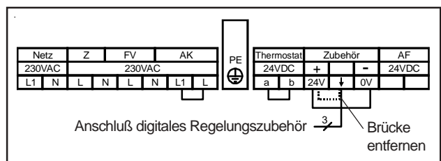
Bild: Anschluß Wolf-Regelungszubehör analog
