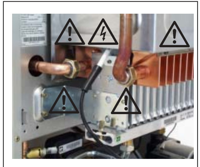
Bild: Hochspannungs-Züdelektrode, Brenner, Brennkammer und Verrohrung Gefahr durch elektrische Spannung, Gefahr von Verbrennung durch heiße Bauteile
