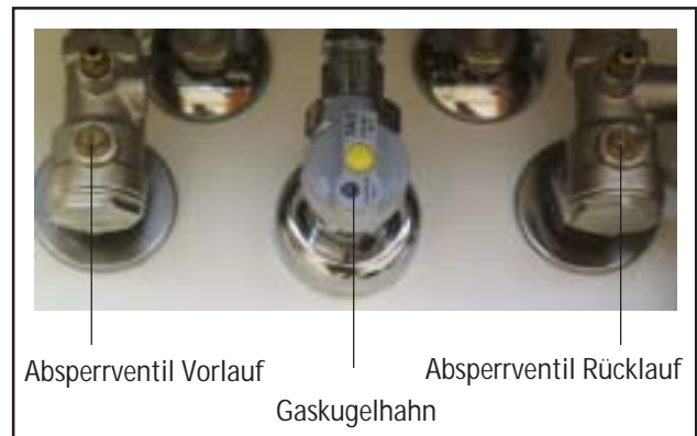
Bild: Absperrreinrichtungen
