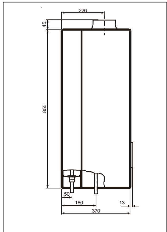
Bild: Abmessungen GU-2E-S
