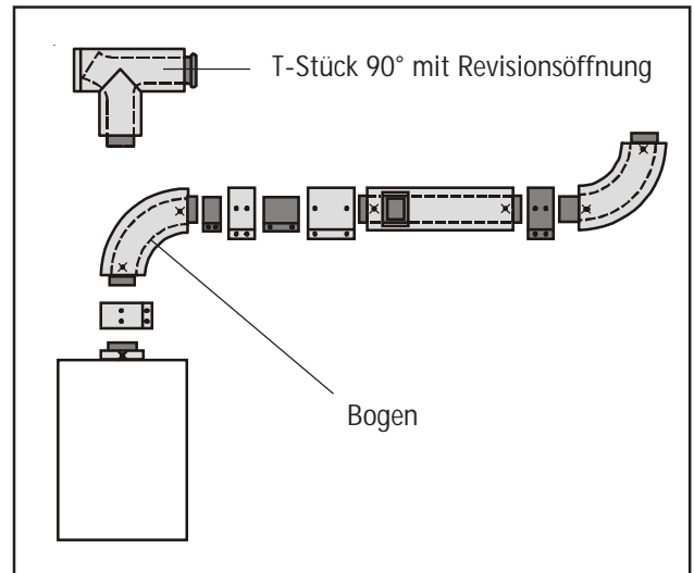
Bild: Rohrlängenberechnung
