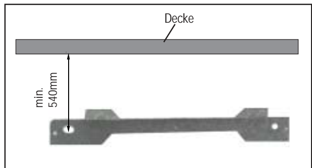
Bild: Bohrlöcher für Einhängewinkel
