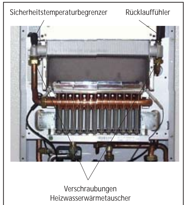
Bild: Demontage Heizwasserwärmetauscher
