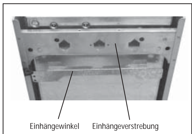
Bild: Gastherme in Einhängewinkel einhängen
