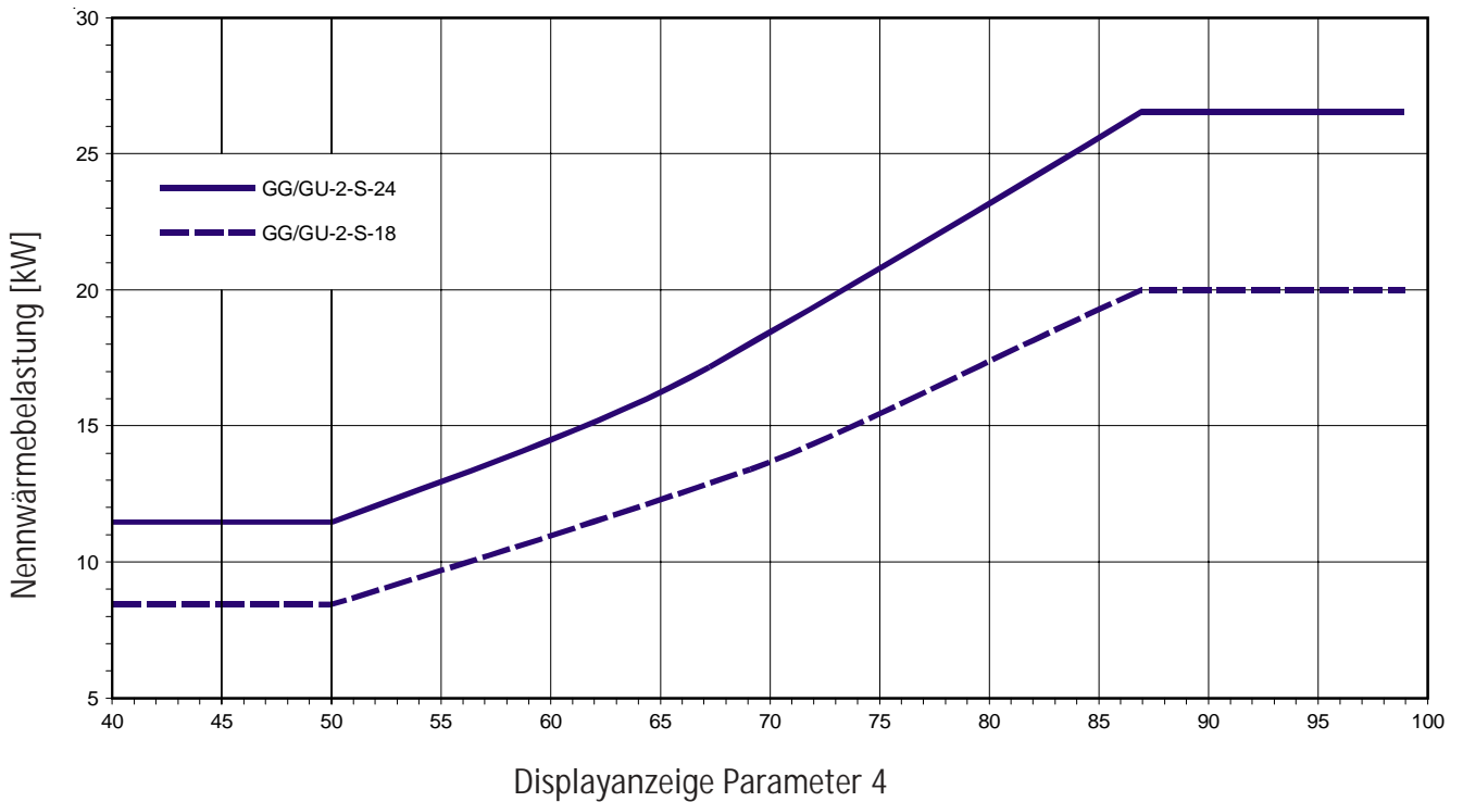
Diagramm: Nennwärmebelastung
