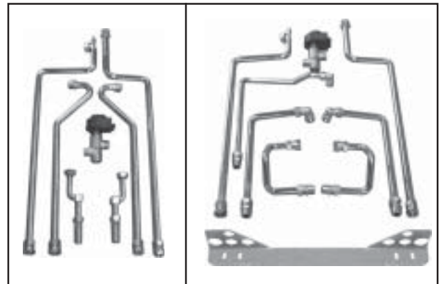
Bild: Anschlußset für Wolf-Speicher 115 Ltr. Unterputzinstallation (Zubehör)
