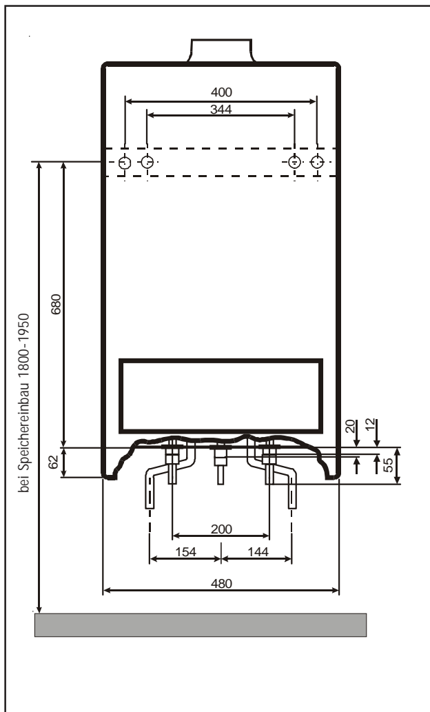
Bild: Abmessungen GU-2E-S
