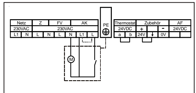
Bild: Anschluß Abgasklappe
